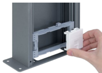
Горизонтальный монтаж
